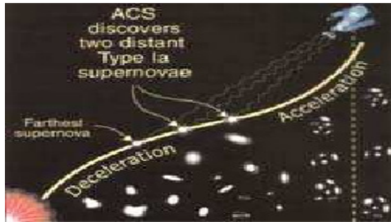
► Малюнок, що ілюструє розширення Всесвіту.
