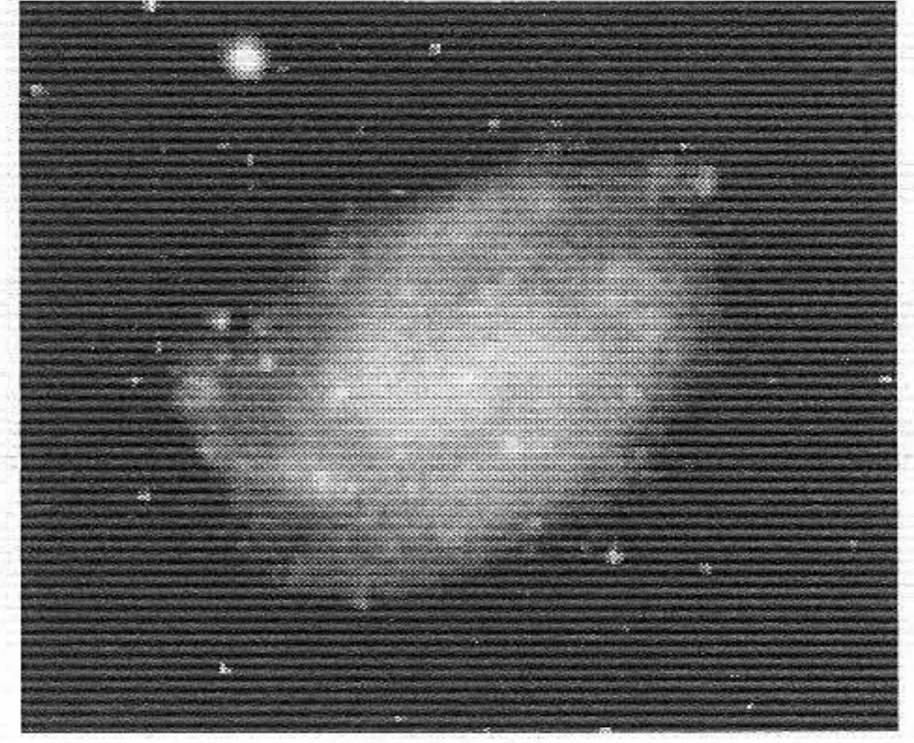
Spiralna galaksija NGC300 u sazviježđu Kipar
