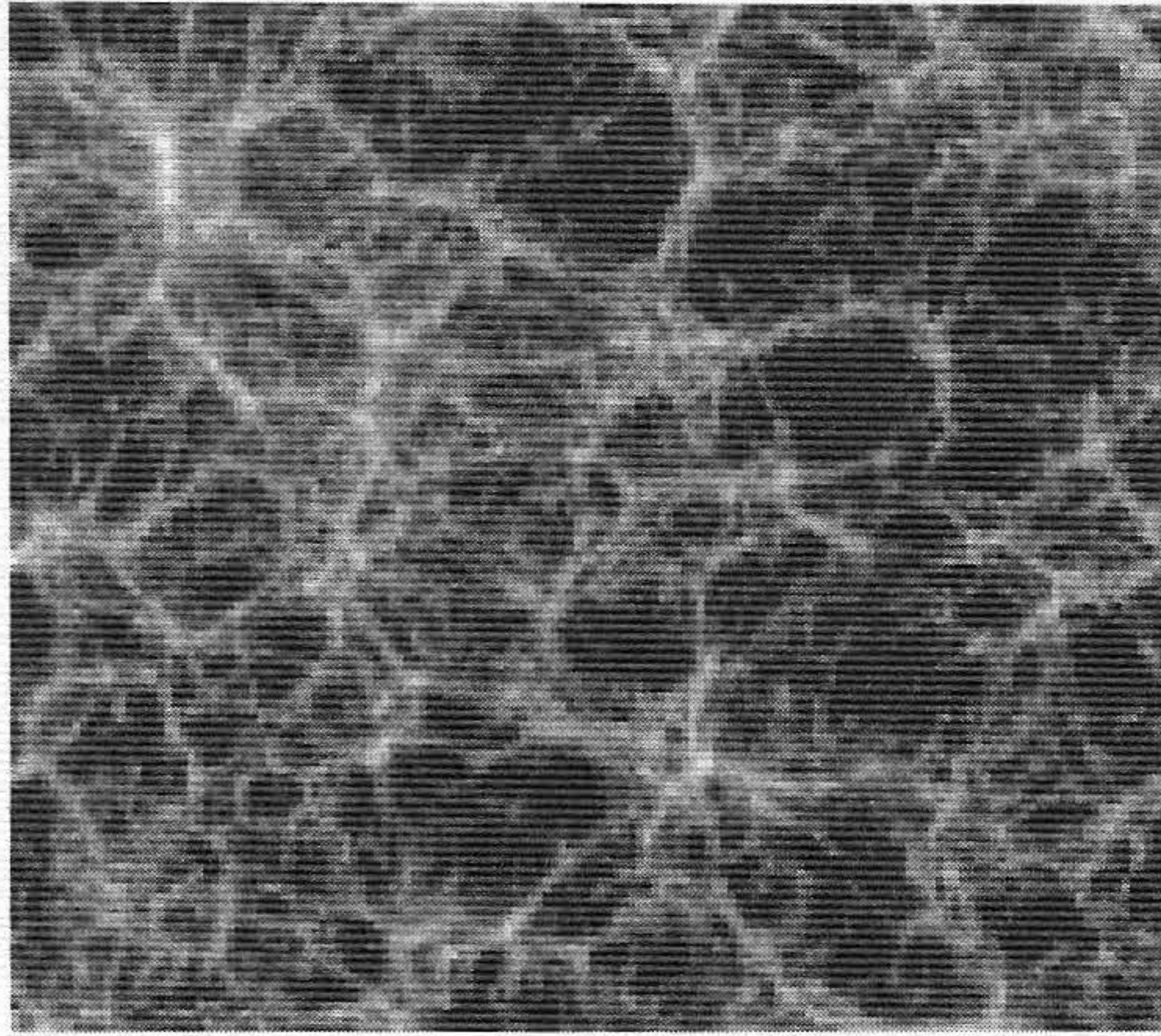
Prve galaksije
