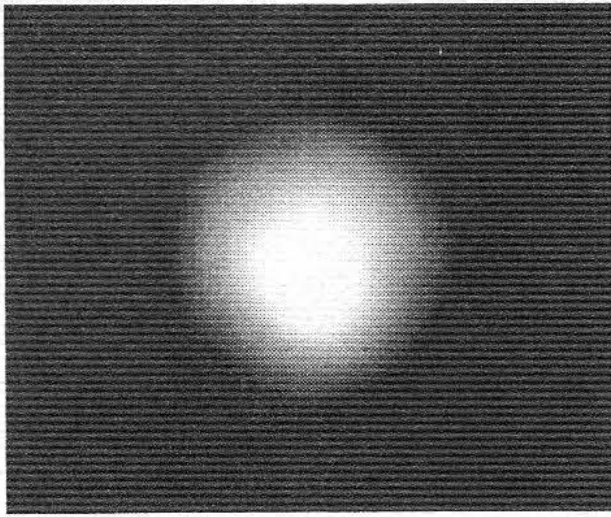
Zvijezda Betelgeuse u Orionu 1000 je puta veća od Sunca (HST)
