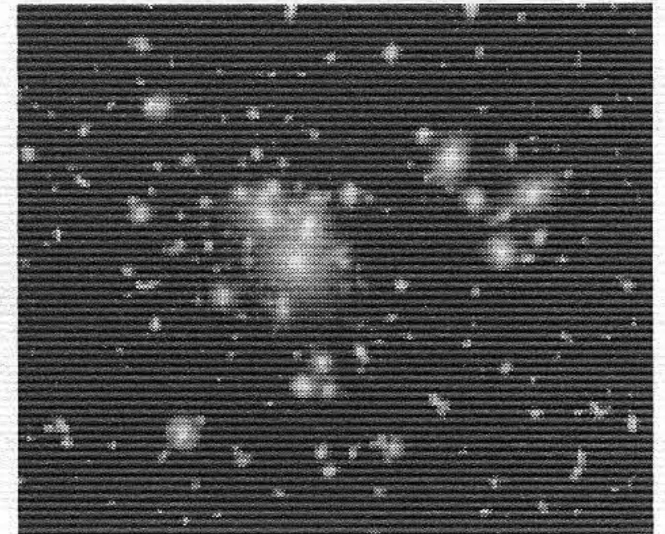
Skup galaksija Abell1689 u sazviježđu Djevica udaljen je 2 milijarde s.g. Skupovi galaksija
