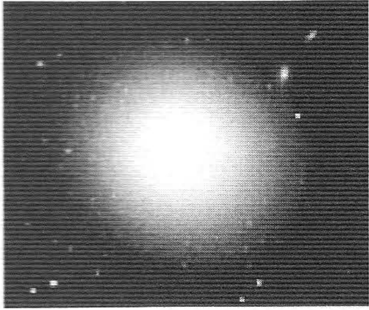
Eliptična galaksija M87 i daleke galaksije u .(pozadini (Anglo-Australian Telescope
