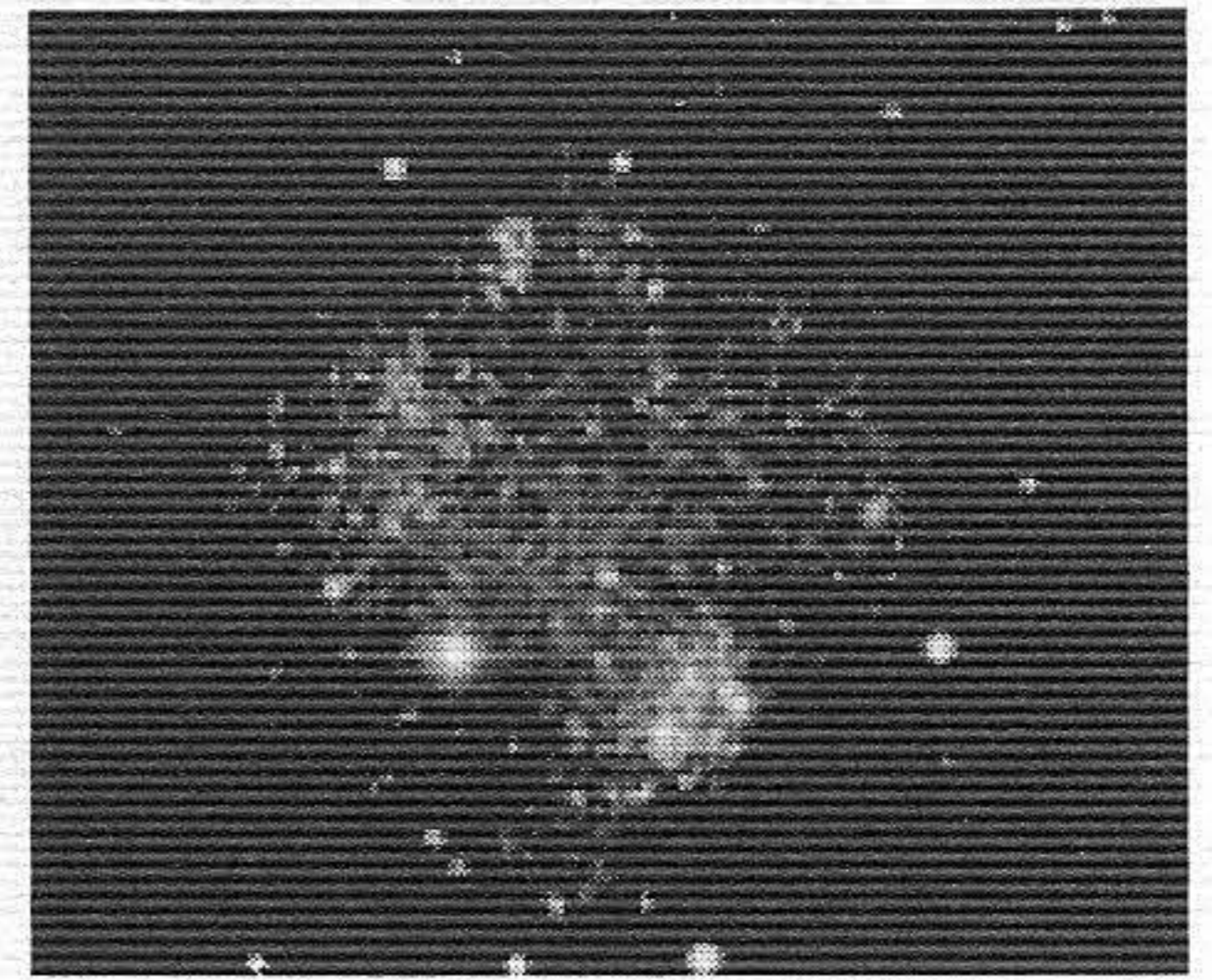
Nepravilna galaksija Sekstant A u sazviježđu Sekstant
