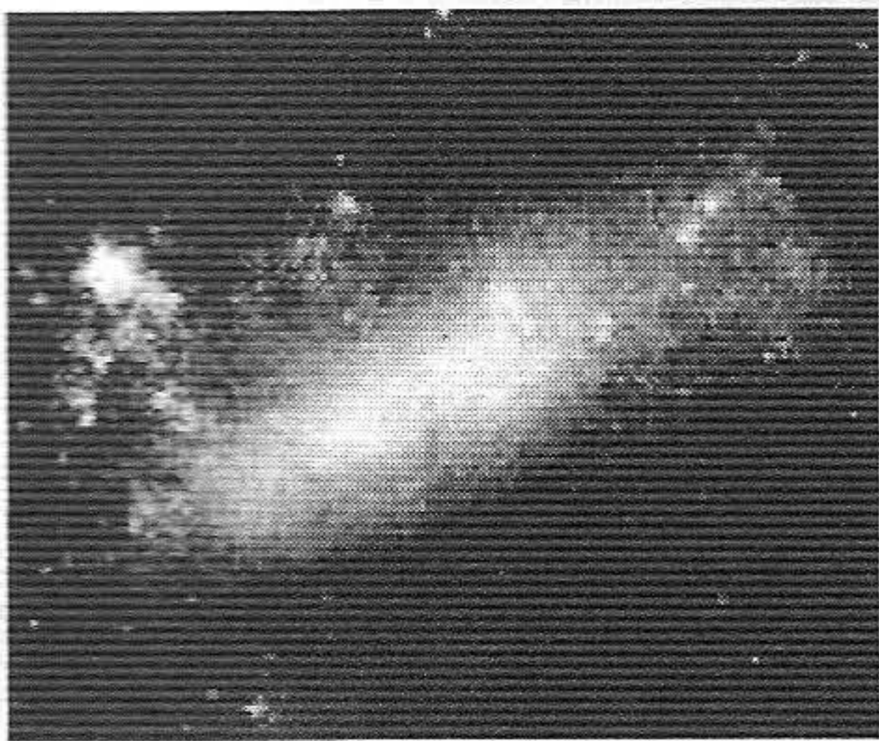
Nepravilna galaksija Veliki Magelanov oblak satelit je Mliječnog puta
