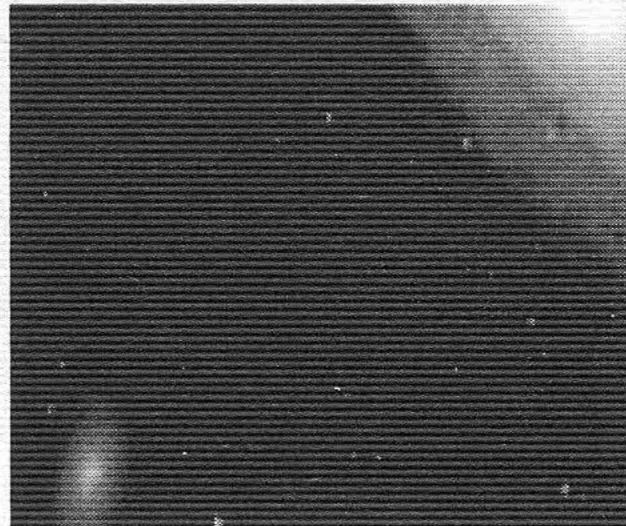
Patuljasta eliptična galaksija M110 satelit je mnogo veće M31 (Andromedina)
