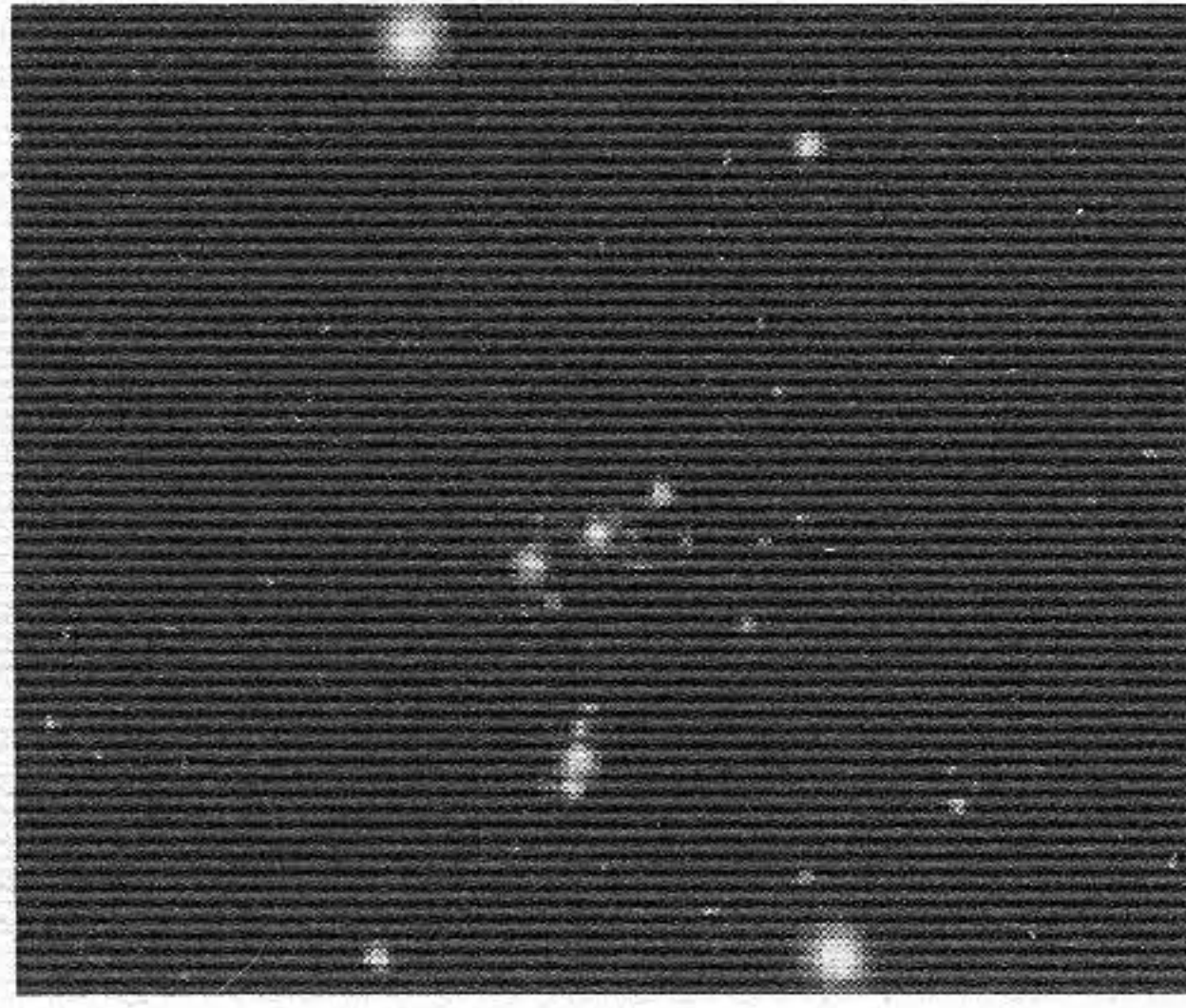
Sazviježđe Orion
