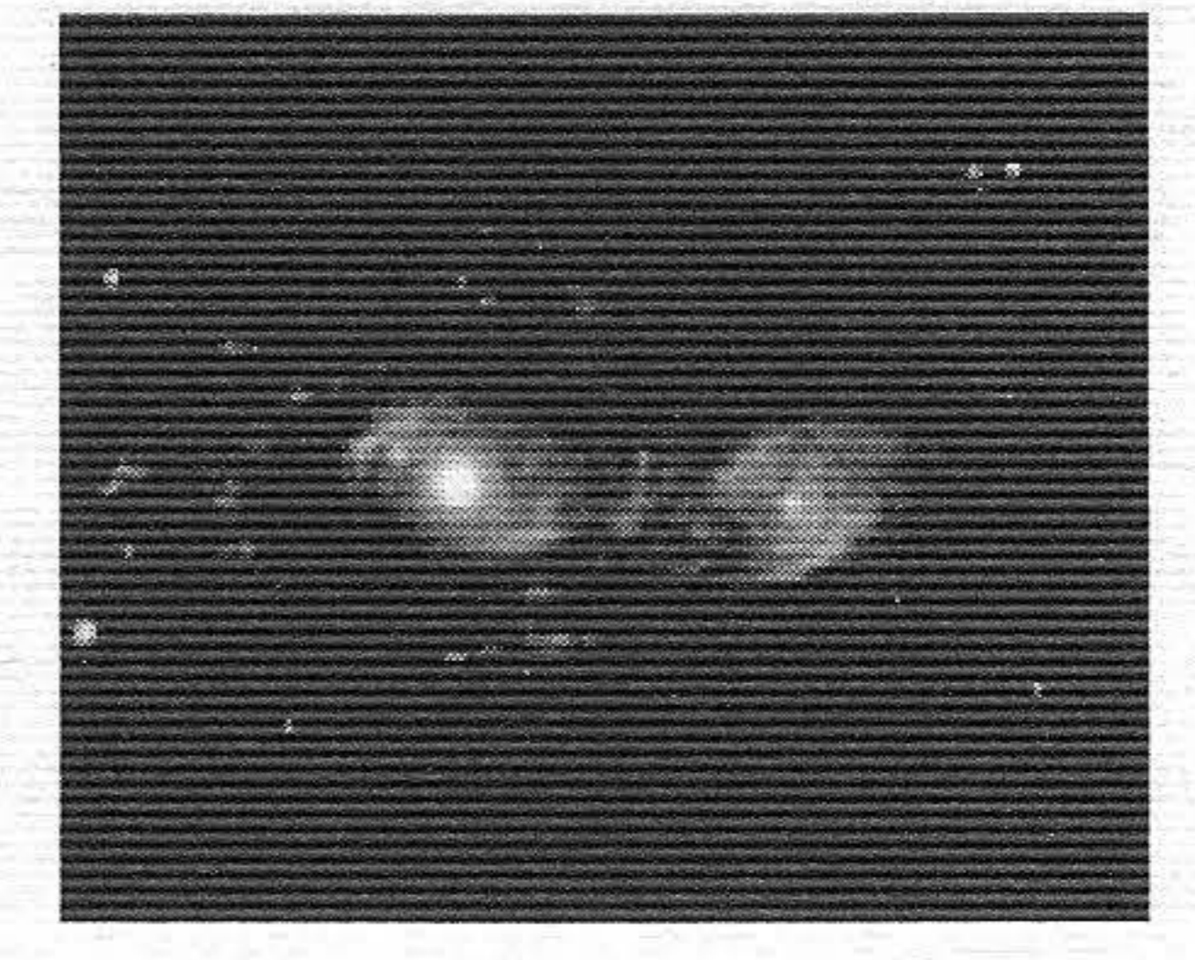
Sudar spiralnih galaksija NGC2207 i IC2163.
