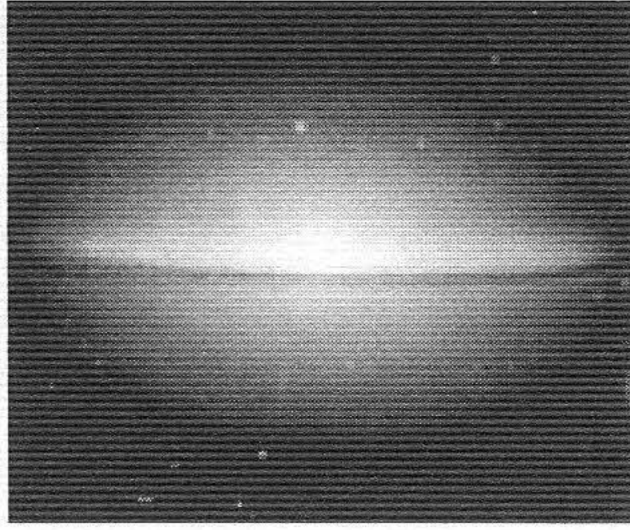
Sočivasta galaksija Sombrero (M104) .udaljena je 50 miliona s.g
