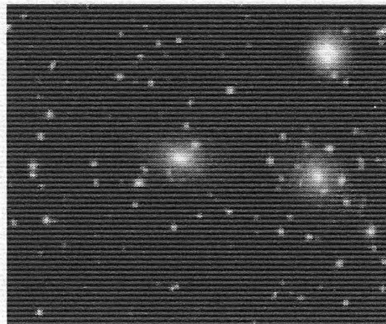
Skup galaksija Coma u sazviježđu Berenikina kosa (Come Berenices). Skupovi galaksija
